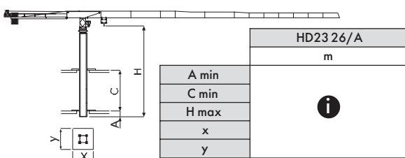
Телескопический кран
